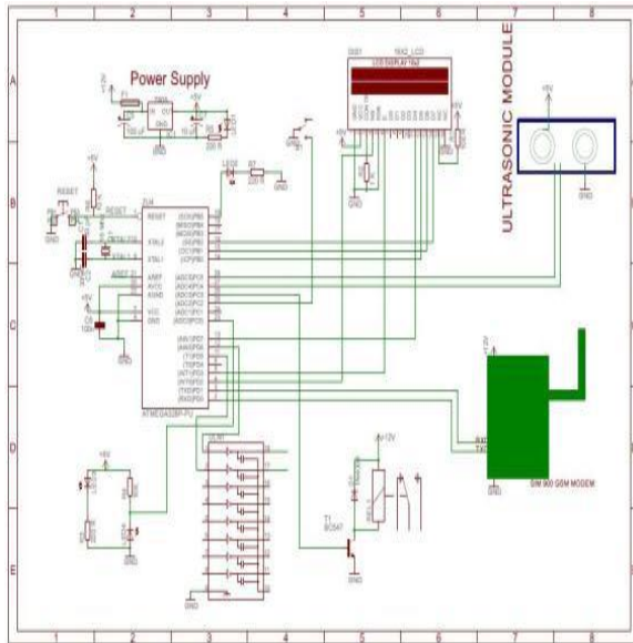
Fig 4: The Actual Circuit
